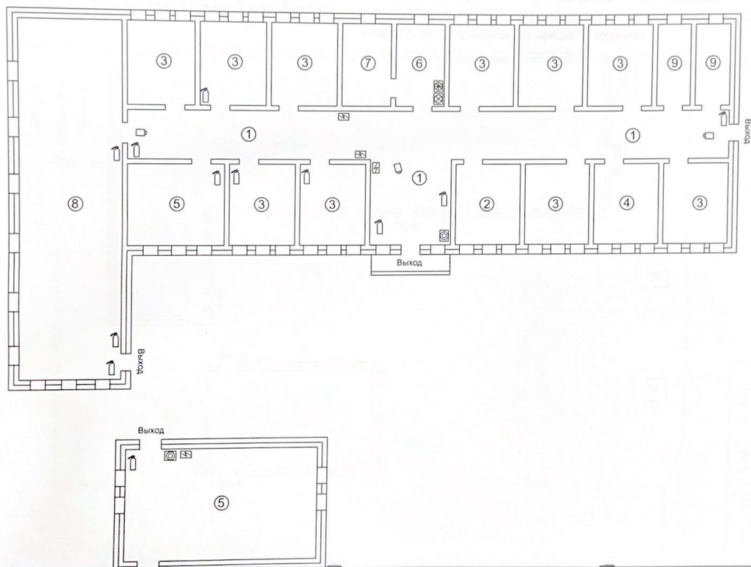
МБОУ "СОШ с. Итум-Кали им.Исаева Х.А. Итум-Калинского муниципального района" План (схема) объекта (территории) с указанием контрольно-пропускных пунктов, постов охраны, инженерно-технических средств охраны.
